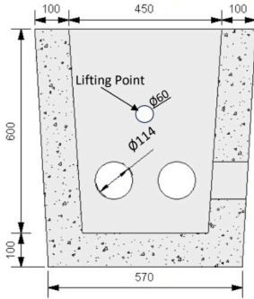
END ELEVATION
