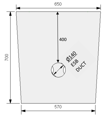
END ELEVATION
